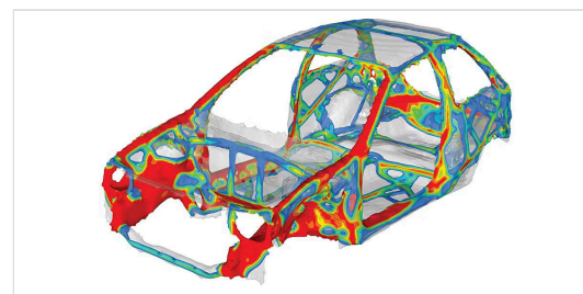
Topologická optimalizace karoserie – OptiStruct hledá tuhou konstrukci s minimem materiálu.
